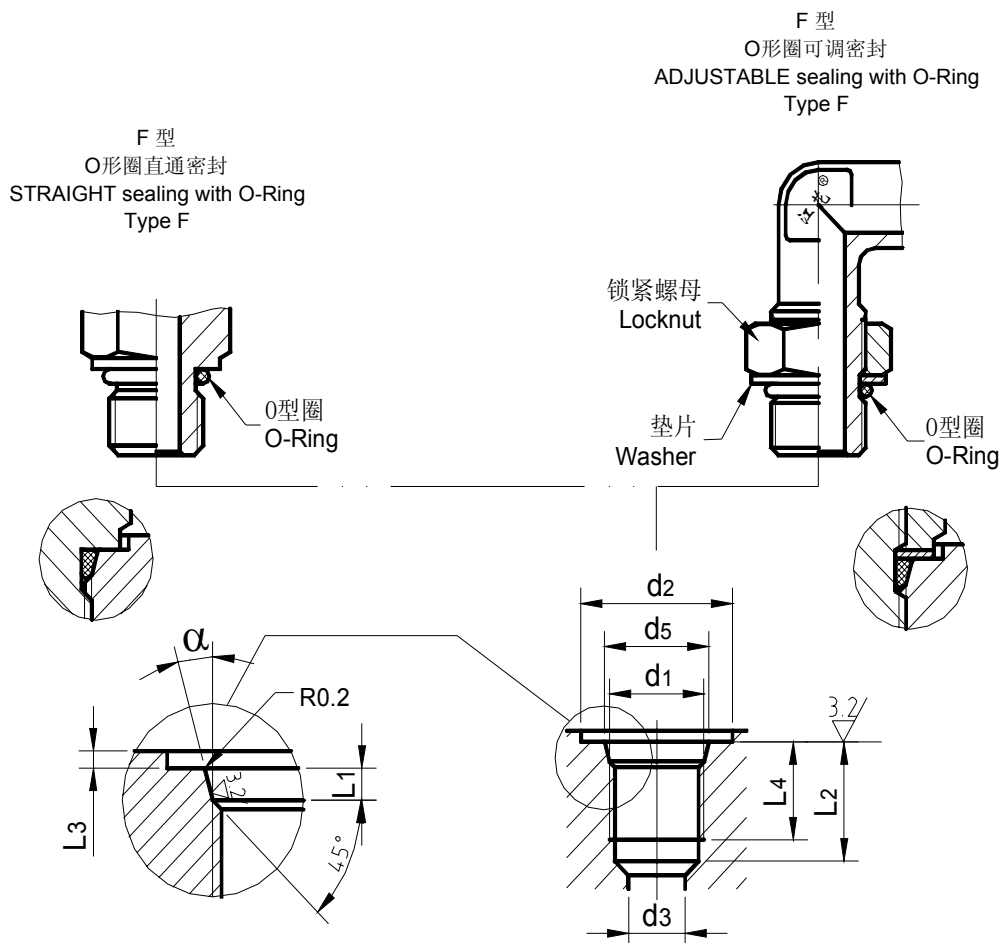
ISO 6149-1 Port Detail
